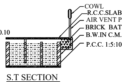
S.T SECTION
