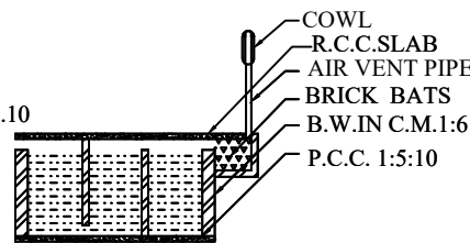
S.T. SECTION
