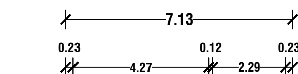
ELEVATION
