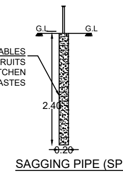
SAGGING PIPE (SP.)
