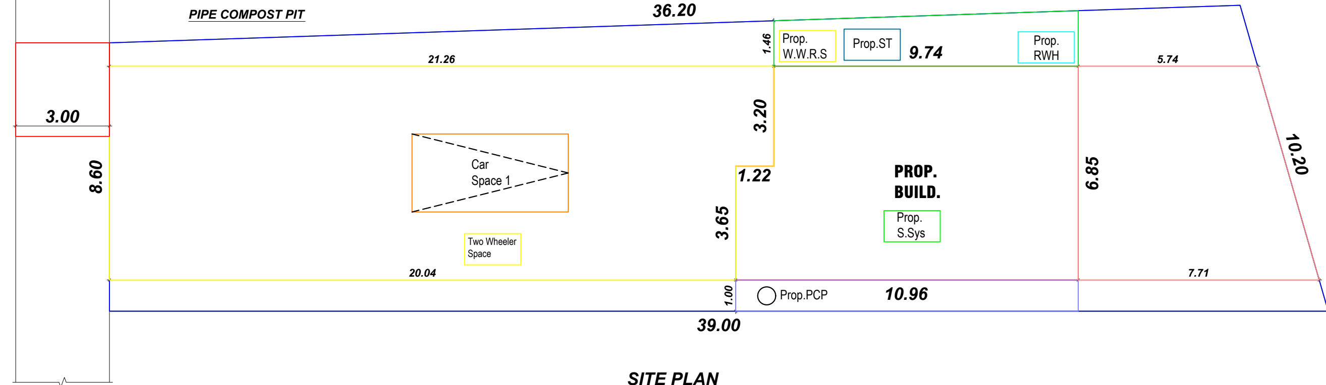
SITE PLAN Scale : 1:100
