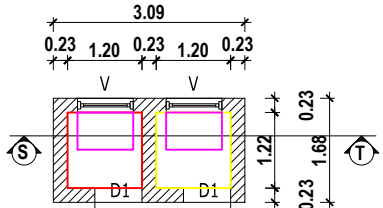
TOILET PLAN
