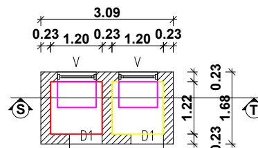
TOILET PLAN
