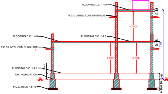
SECTIONN A-A
