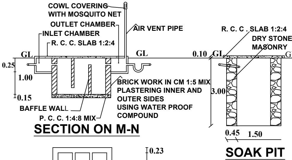
SOAK PIT
