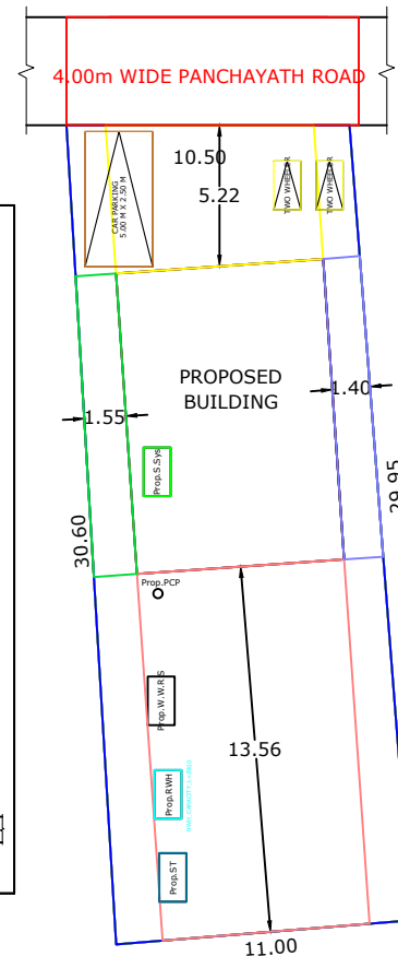
SITE PLAN SCALE - 1:100
