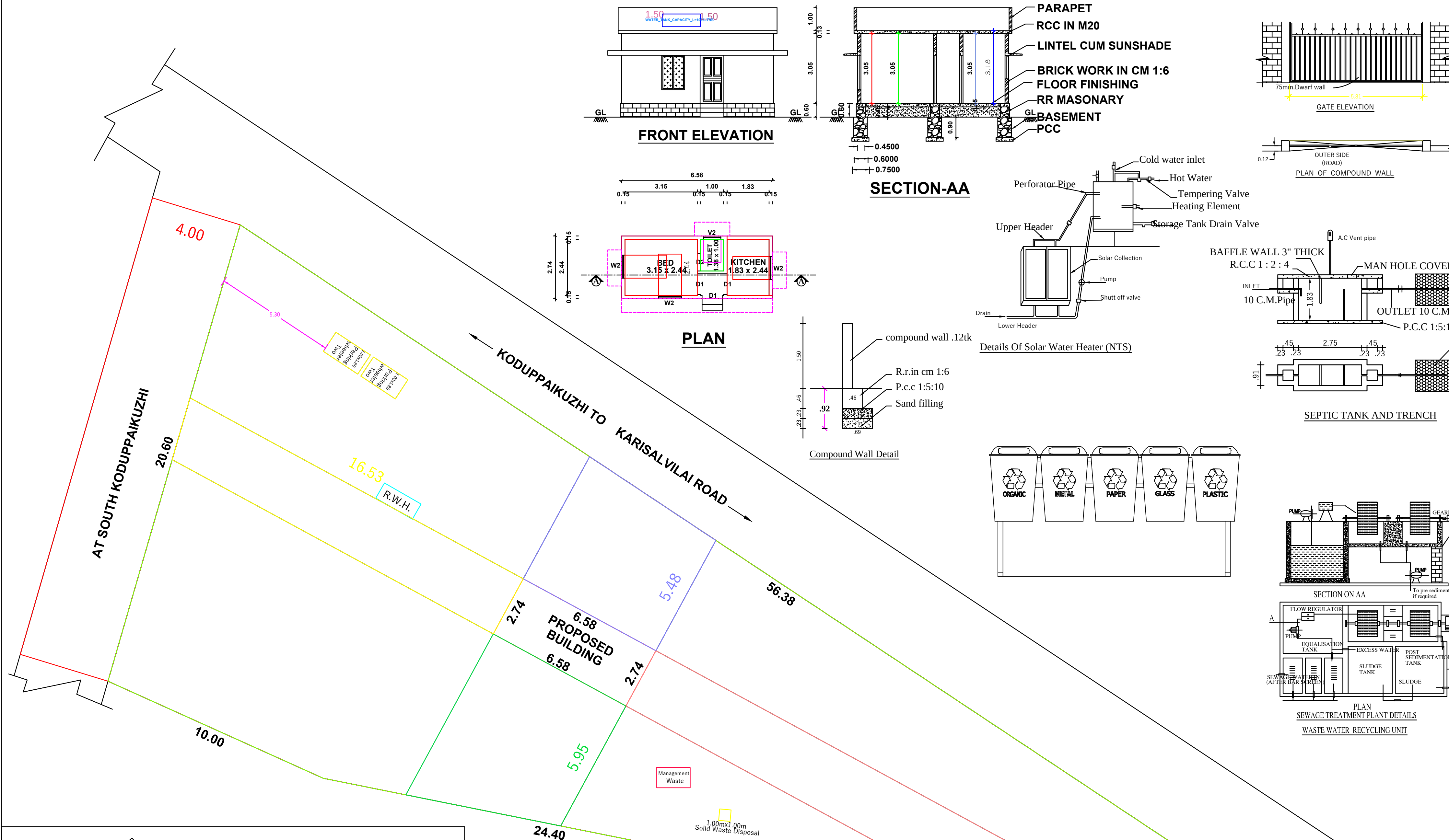
SITEPLAN (SCALE -1:100)
