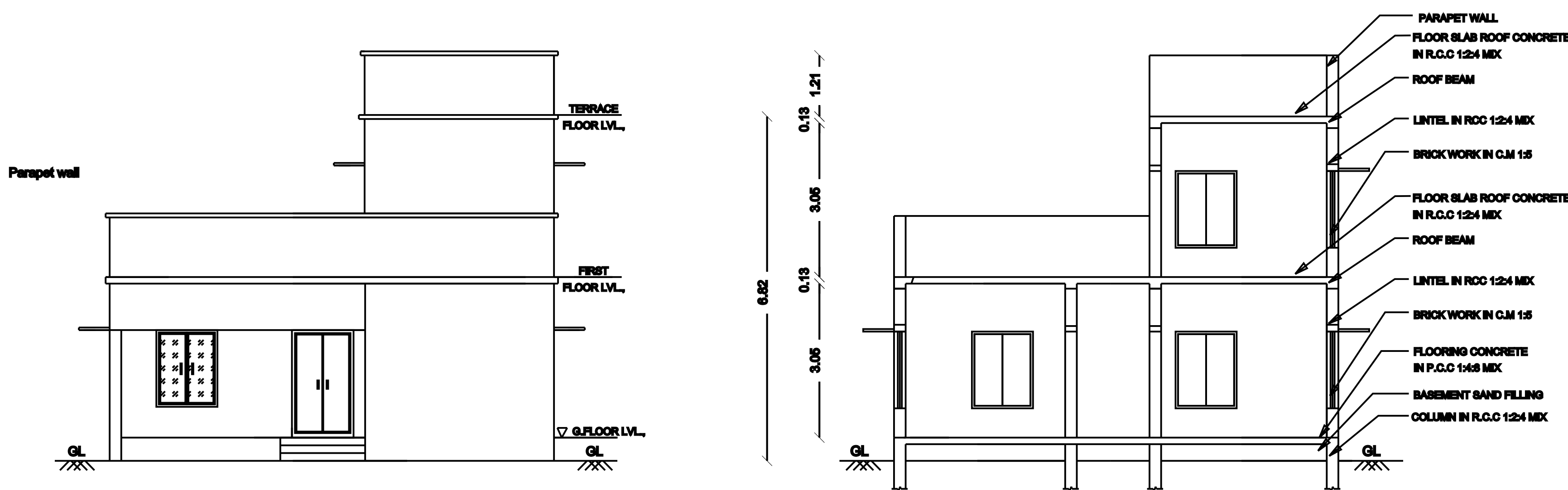
ELEVATION
