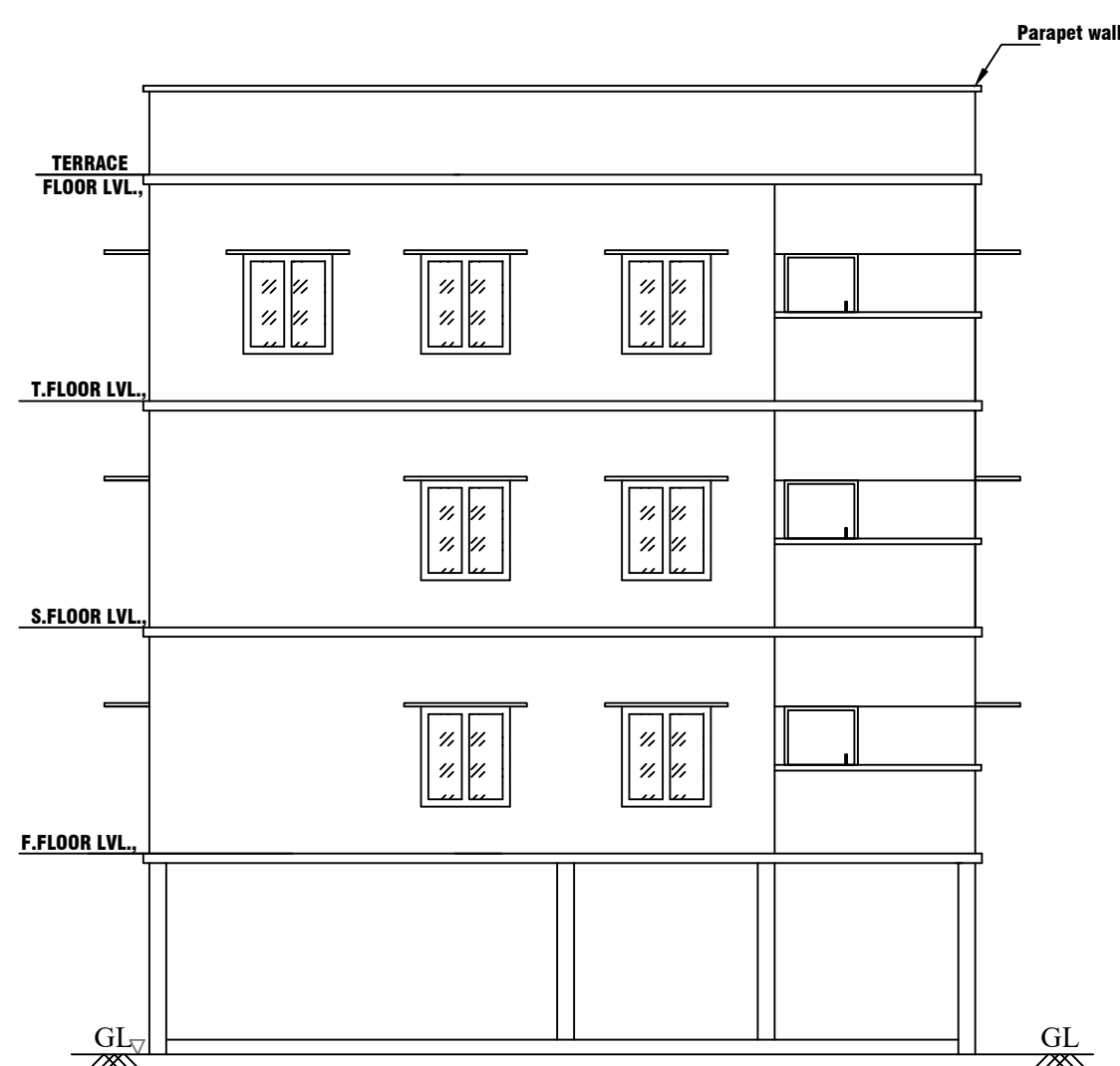
ELEVATION
