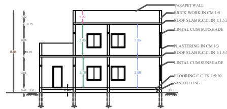
SECTION NO A-A
