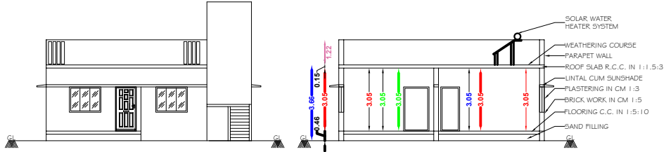
ELEVATION
