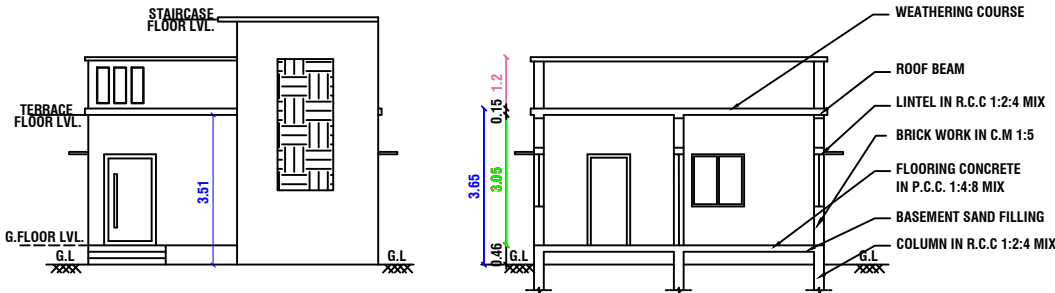
ELEVATION
