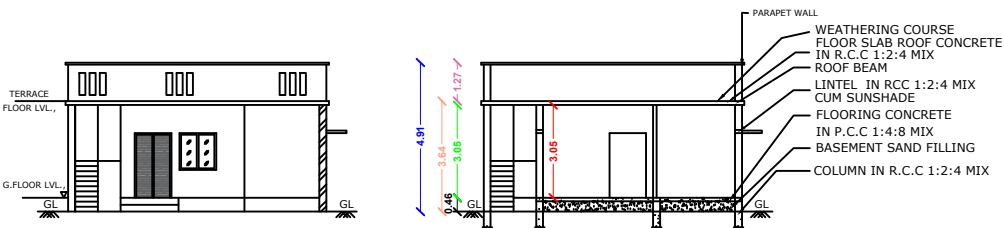
ELEVATION
