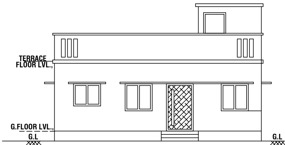
ELEVATION
