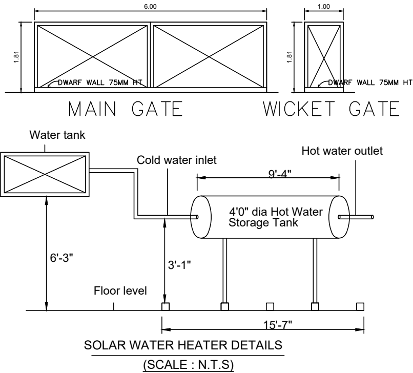
SOLAR WATER HEATER DETAILS (SCALE : N.T.S)
