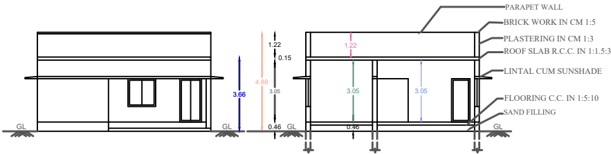
ELEVATION
