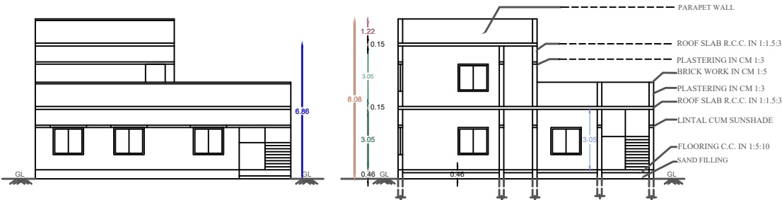
ELEVATION
