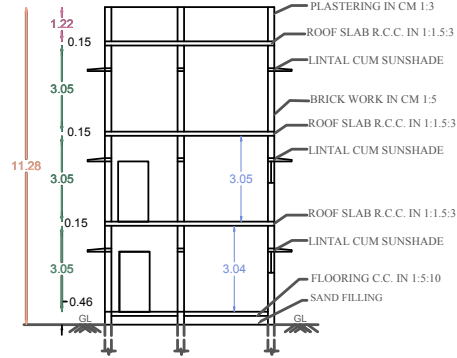
SECTION NO A-A
