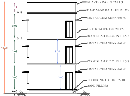
SECTION NO A-A
