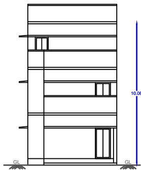
ELEVATION
