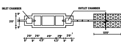
PLAN OF S.P.T & D.T
