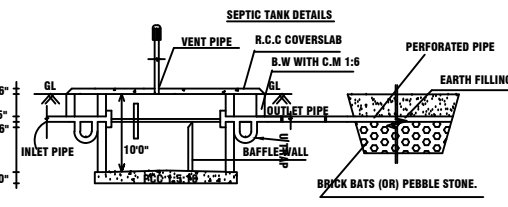
SECTION OF S.P.T & D.T
