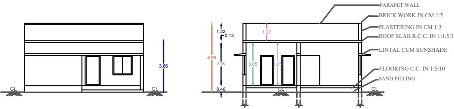
ELEVATION
