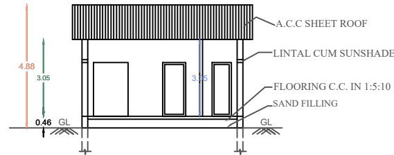
SECTION NO A-A
