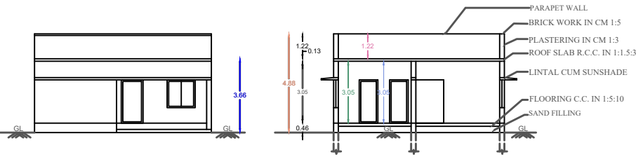
ELEVATION
