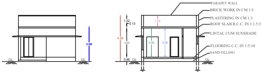
SECTION NO A-A
