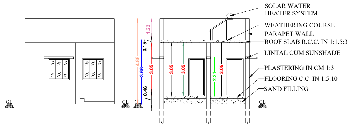
ELEVATION
