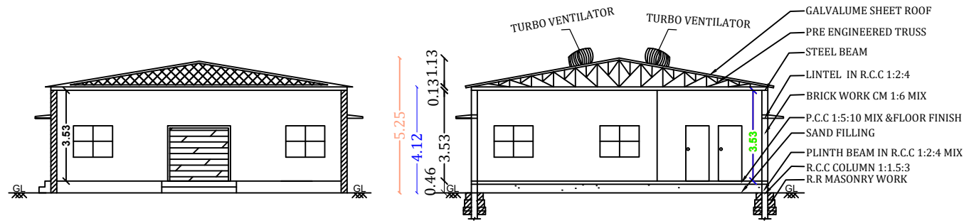
ELEVATION
