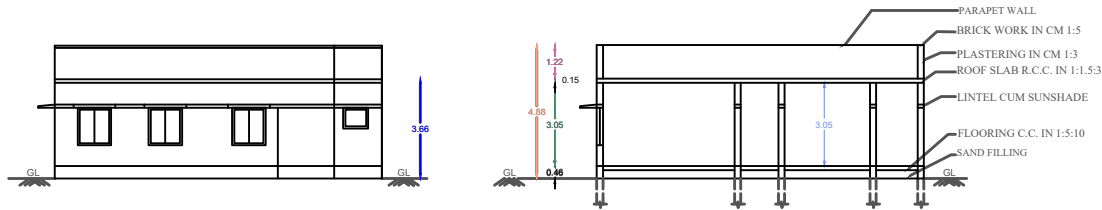
ELEVATION
