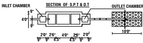
SECTION OF S.P.T & D.T
