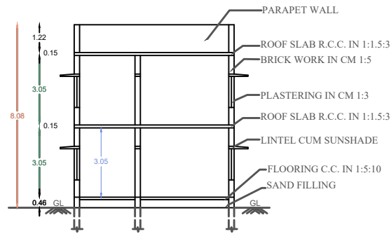
SECTION NO A-A
