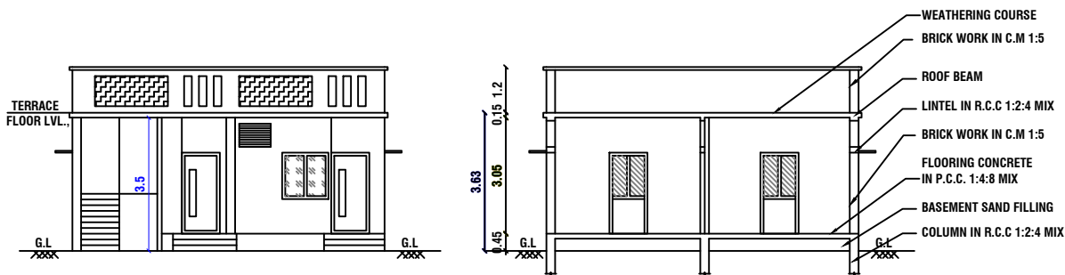
ELEVATION
