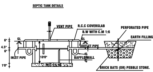
SECTION OF S.P.T & D.T
