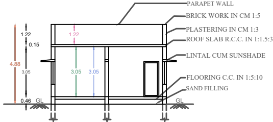
SECTION NO A-A
