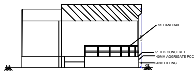
ELEVATION
