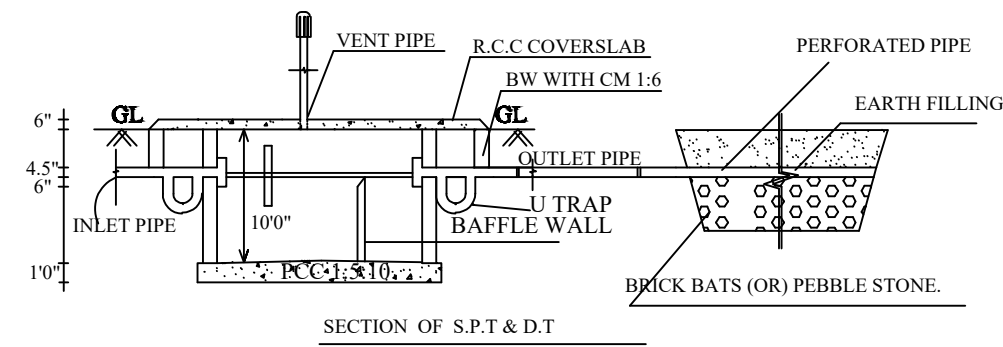
SECTION OF S.P.T & D.T
