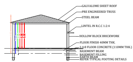
SECTION A-B
