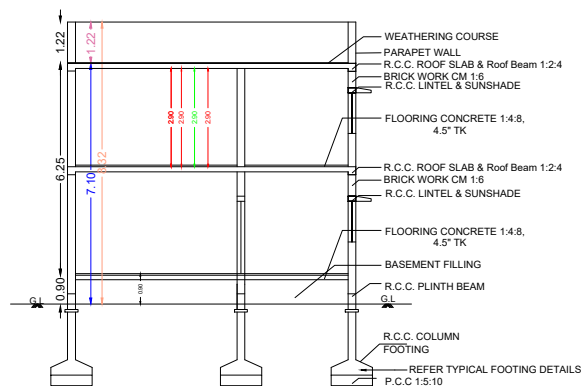
SECTION A-B
