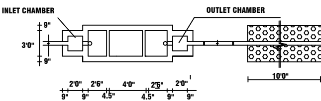
PLAN OF S.P.T & D.T
