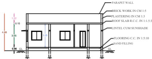
SECTION NO A-A
