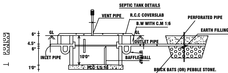
SECTION OF S.P.T & D.T
