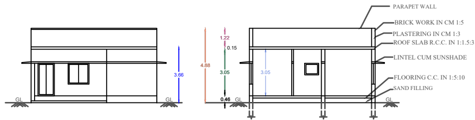
ELEVATION
