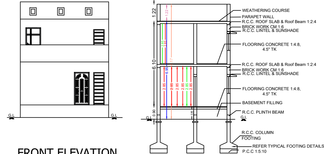
SECTION A-B
