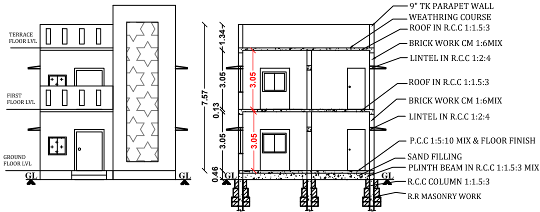
ELEVATION
