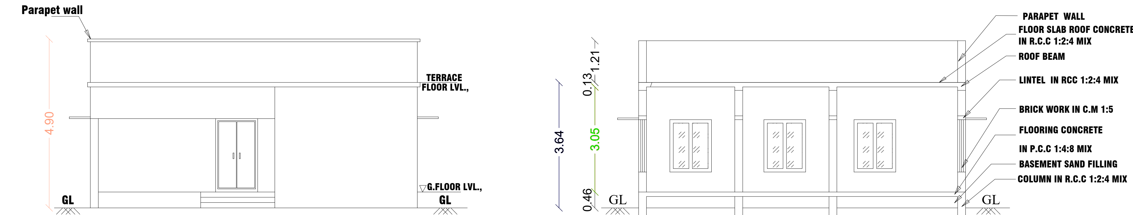
ELEVATION
