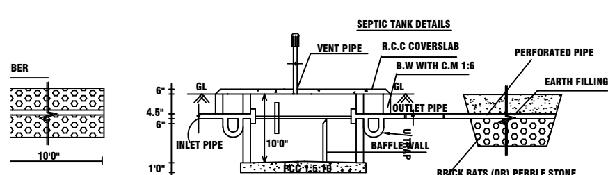
SECTION OF S.P.T & D.T
