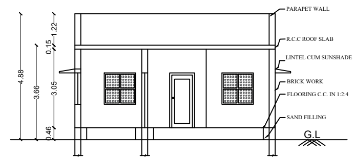
SECTION A-B
