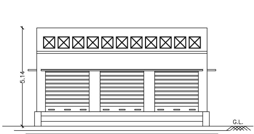
ELEVATION
